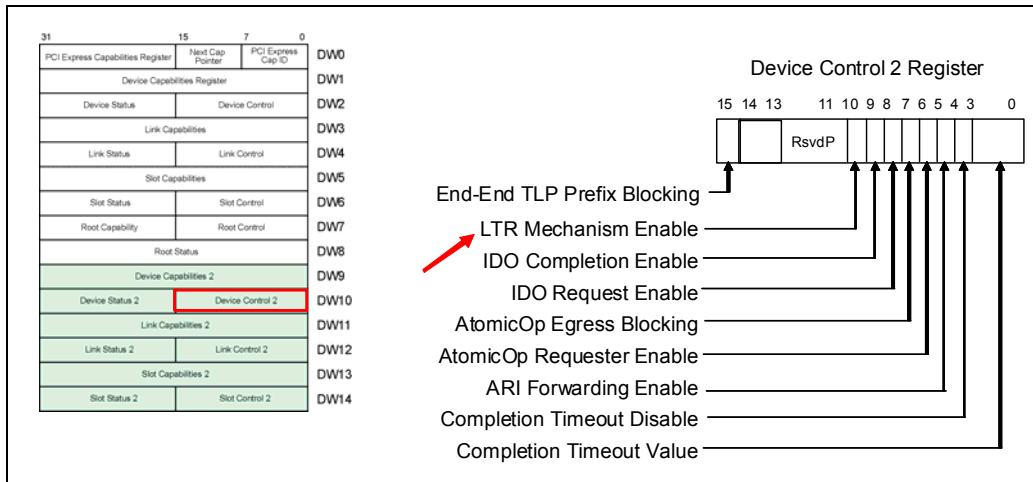
Figure 16-39: LTR Enable
